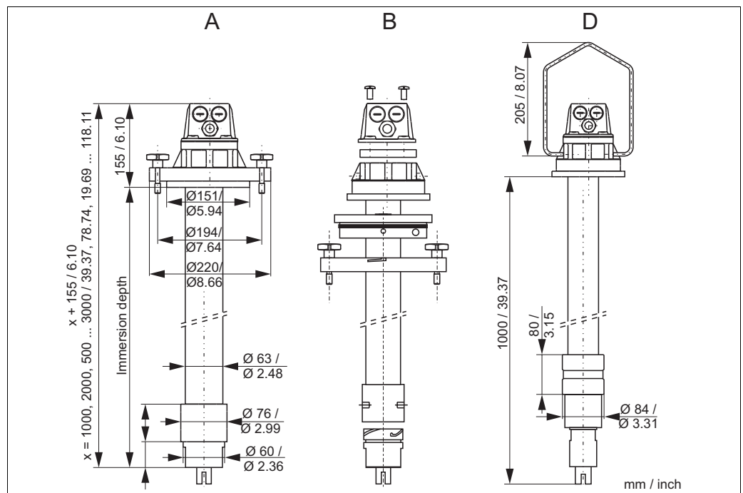
Fig. 42: OLA111, DN 100 flange, mounting versions A, B und D
